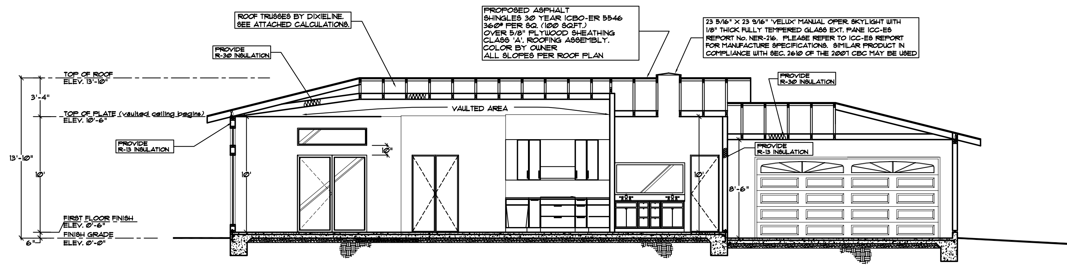
SECTION 4 SCALE: 1/4"=1'-0" A-5
