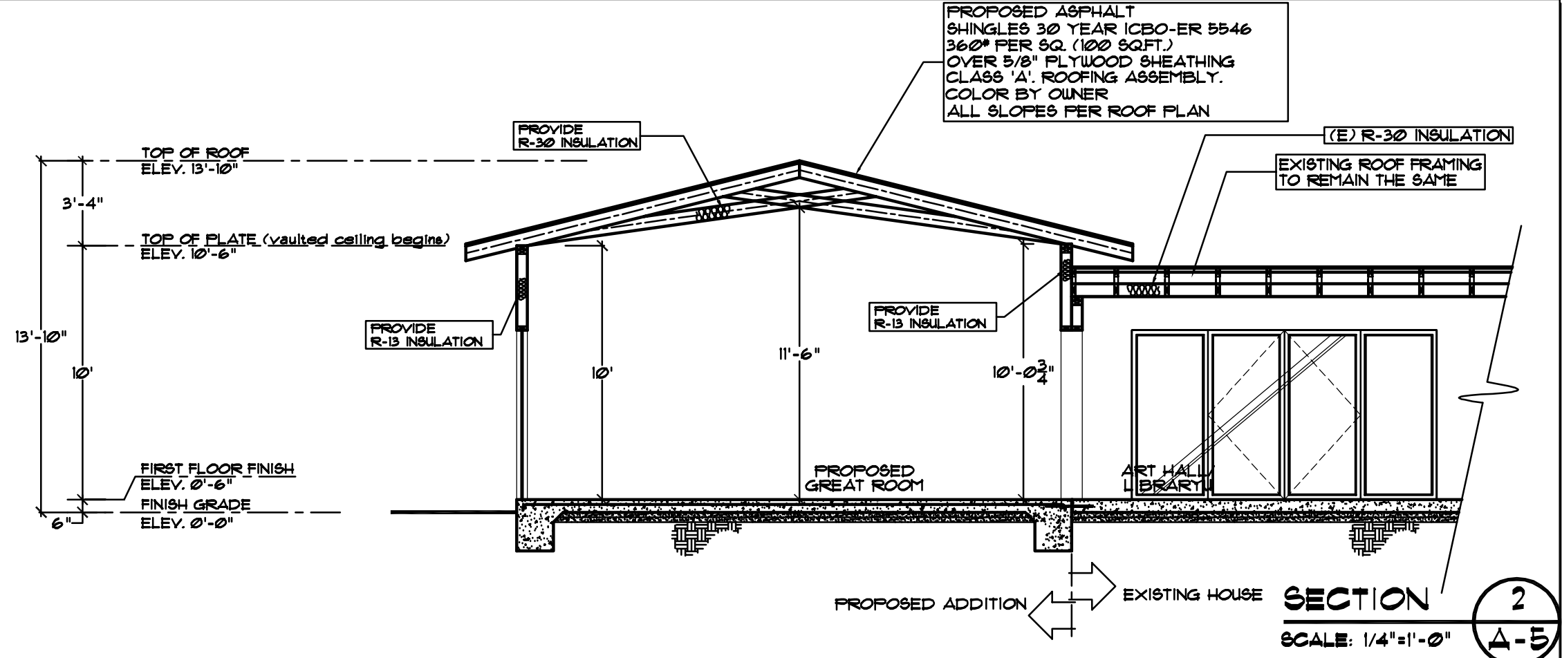
SECTION 1 SCALE: 1/4"=1'-0" A-5
